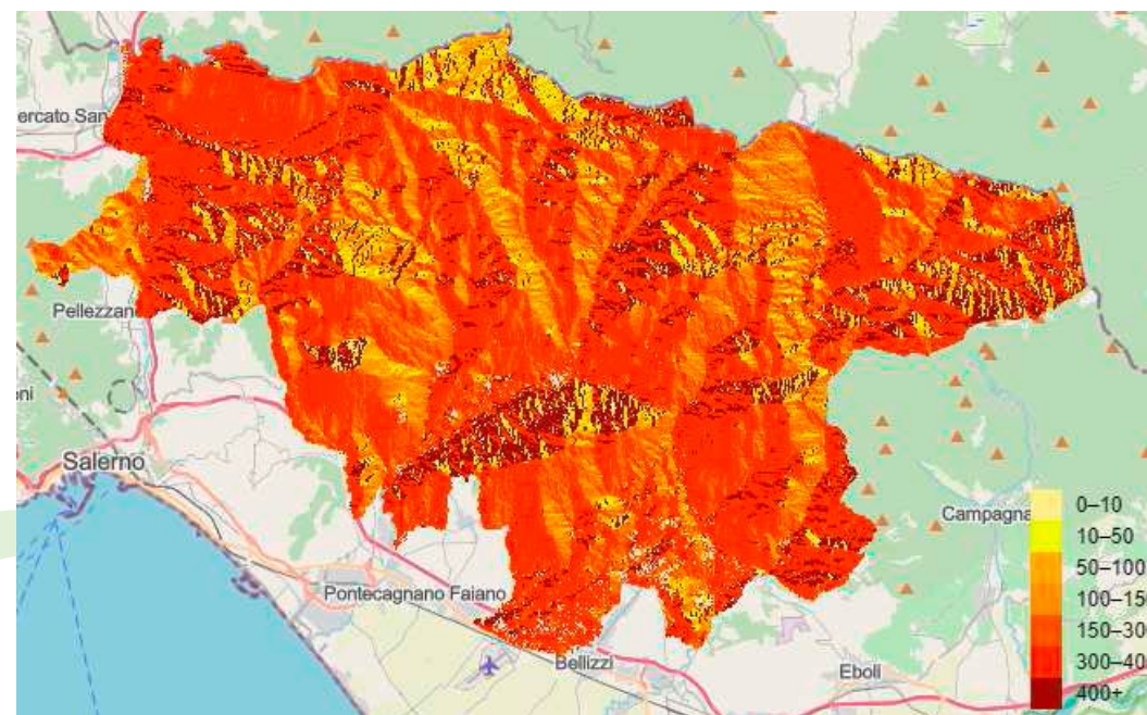
Esposizione solare
