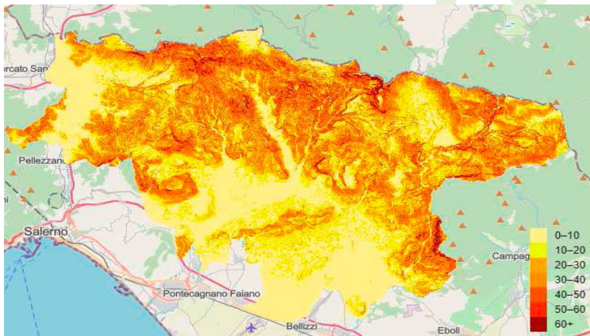
Pendenza
