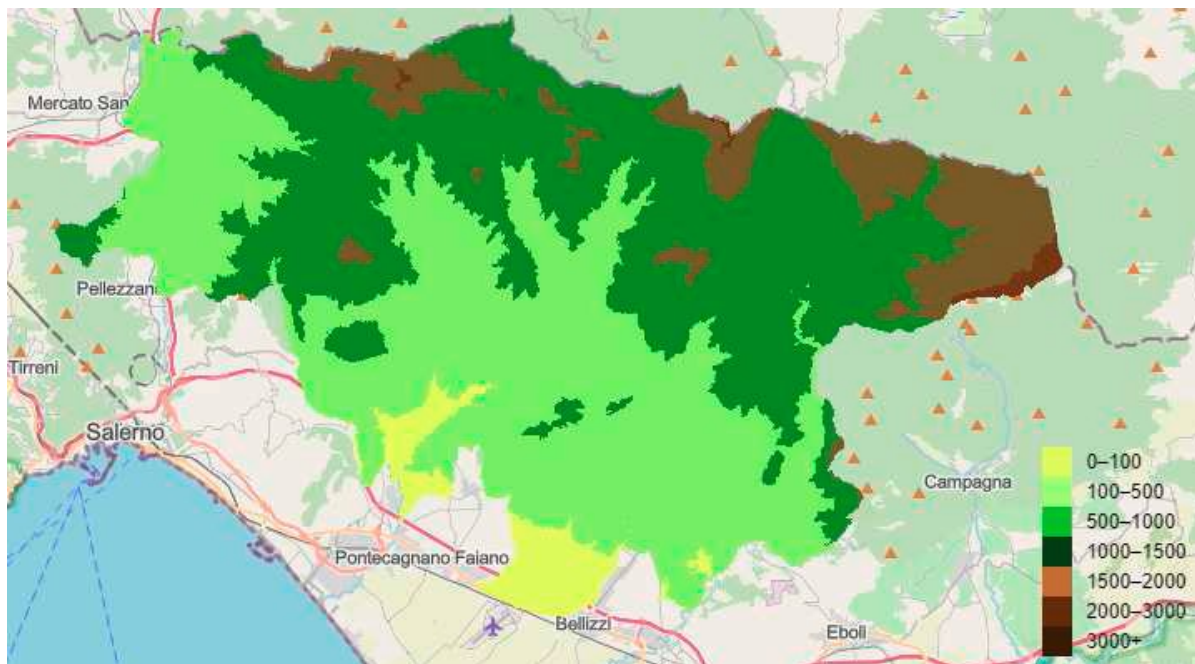
Altitudine (DEM)
